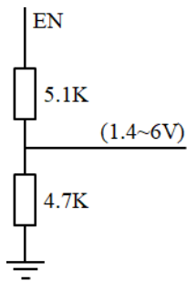
EN circuit on LCM
